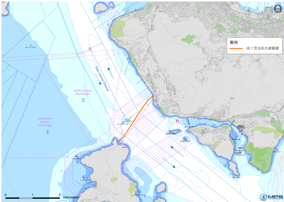
圖 1 - 南丫島海底光纖電纜 (香港鋼綫灣至南丫島北角咀)
