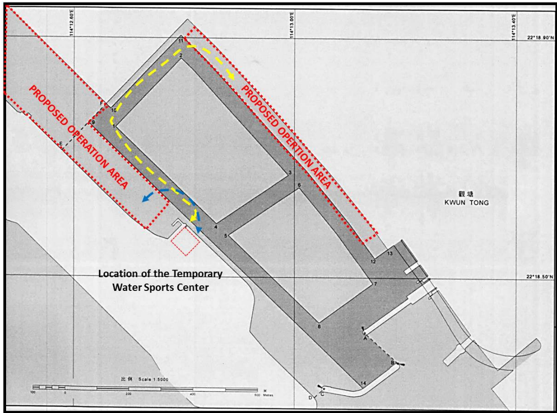
水上活動範圍及由該中心進入該範圍的路線圖
