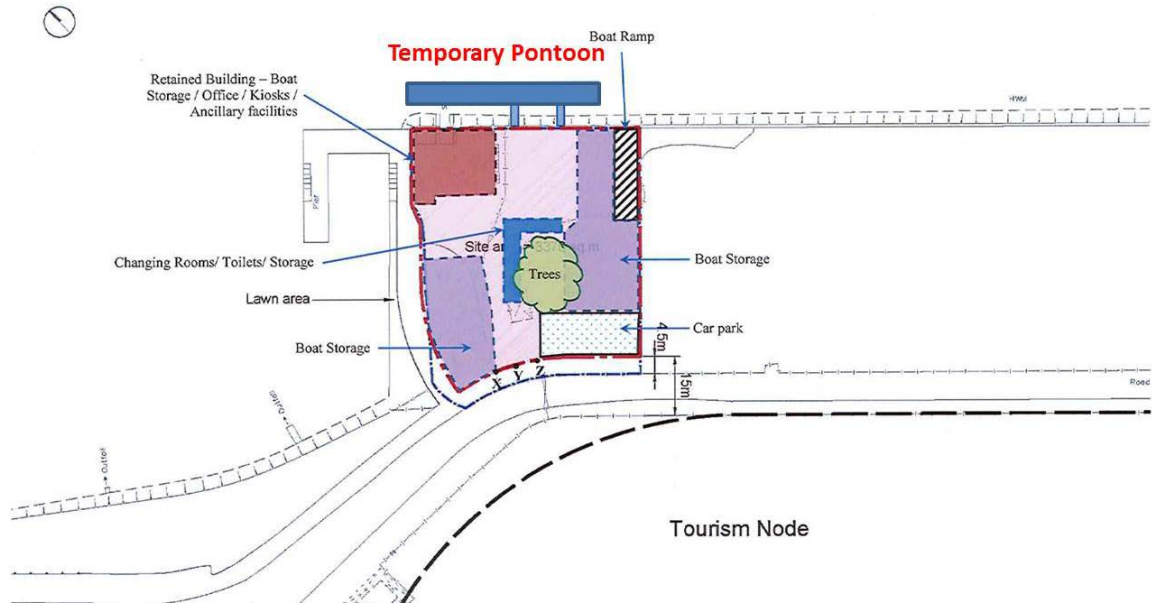
水上活動中心總平面圖
