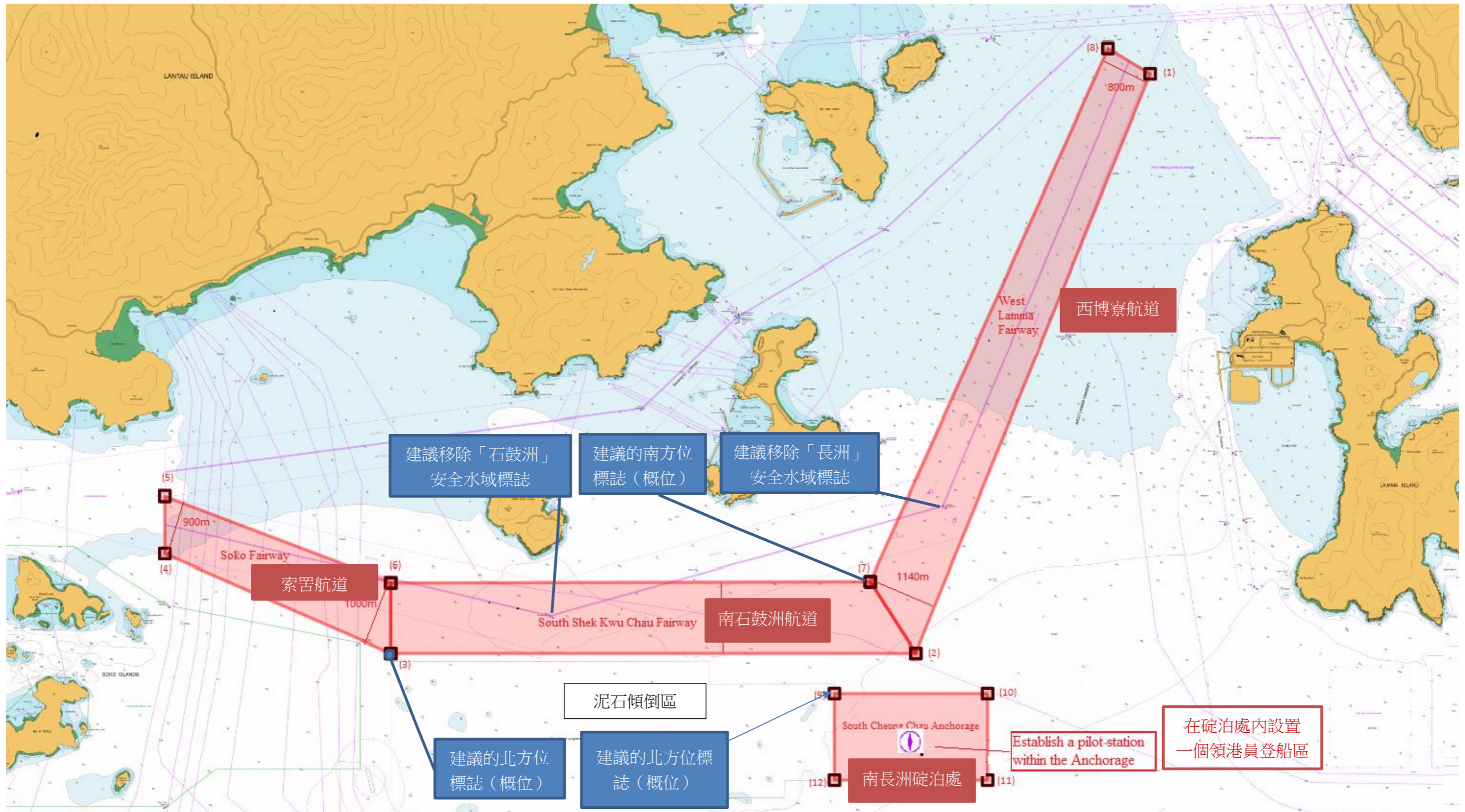
建議新航道系統、新多用途碇泊處（南長洲碇泊處）、新領港員登船區和輔航設備的佈局
